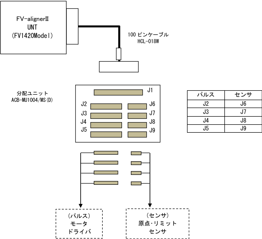
接続コネクタと軸名称
