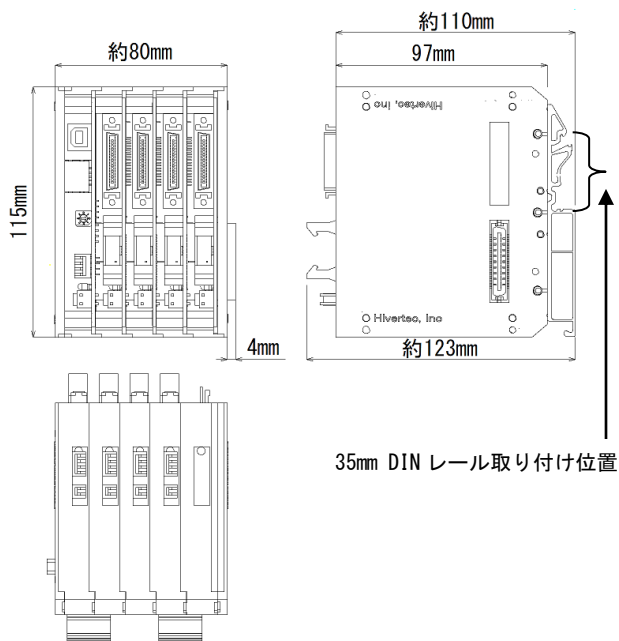
HUG-C4 外形図
