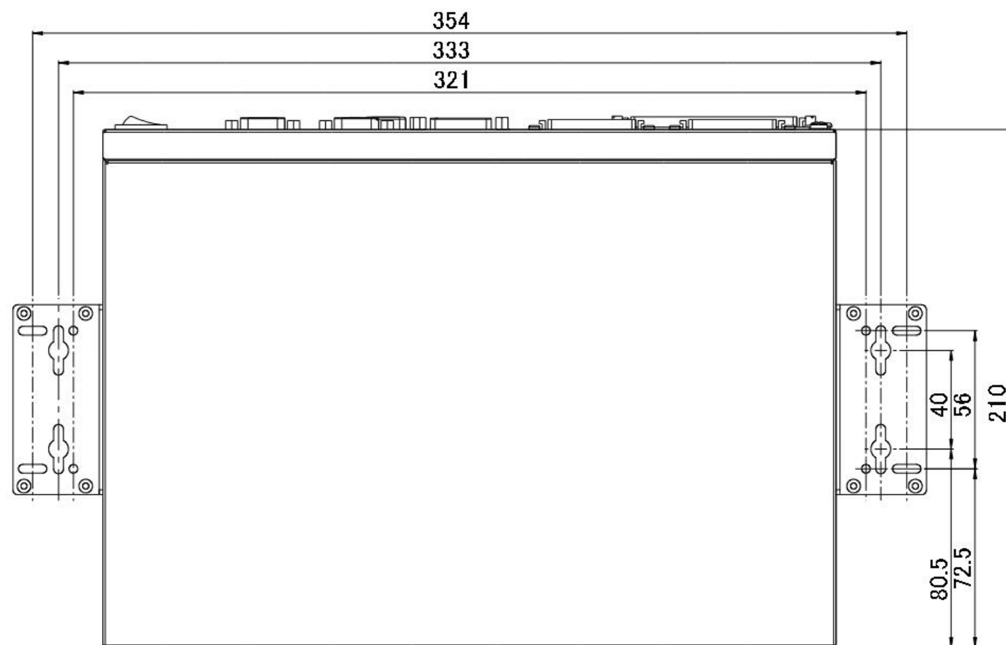
取り付け金具寸法
