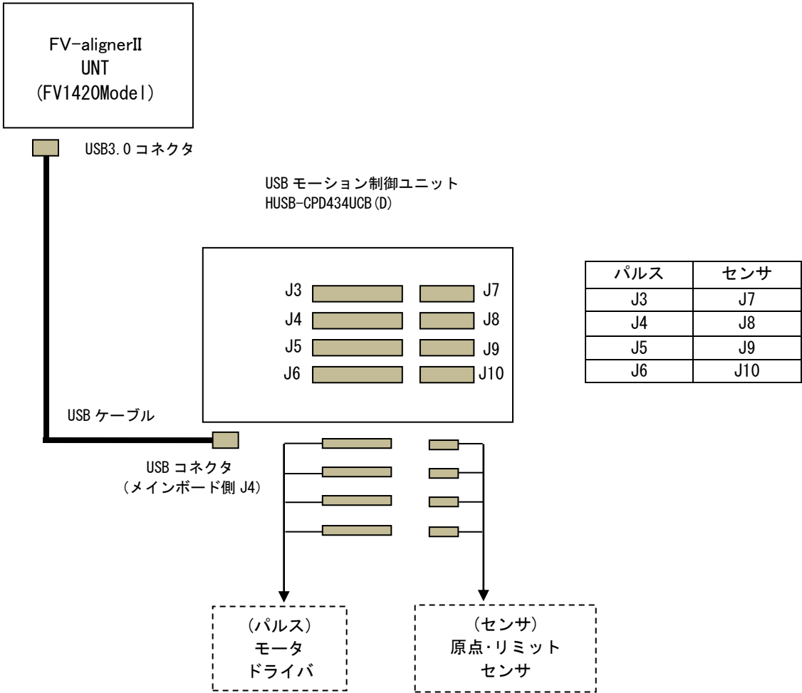
接続コネクタと軸名称
