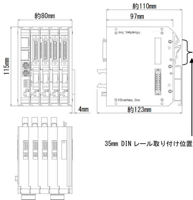
HMG-C4 外形図
