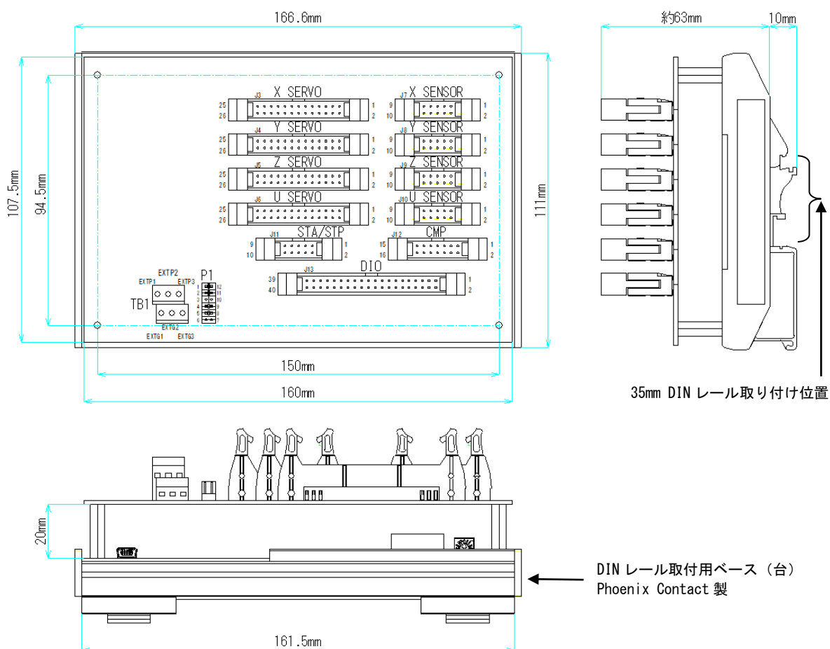
HUSB-CPD434UCB(D) 外形図
