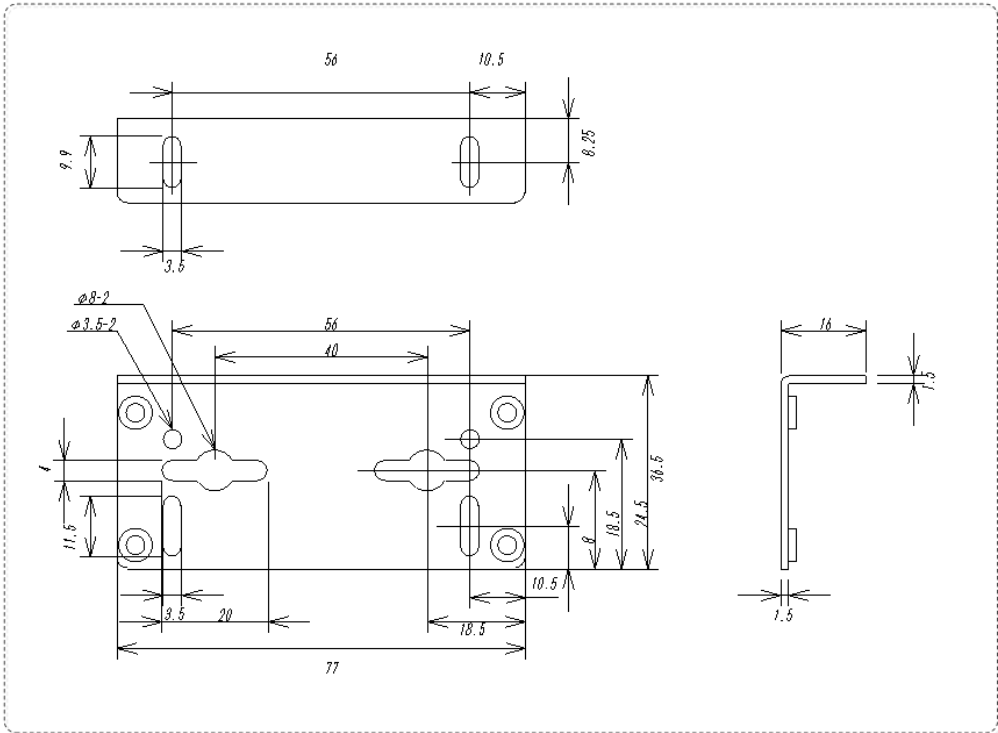
取り付け金具寸法
